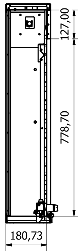
C-C ( 1 : 10 )
